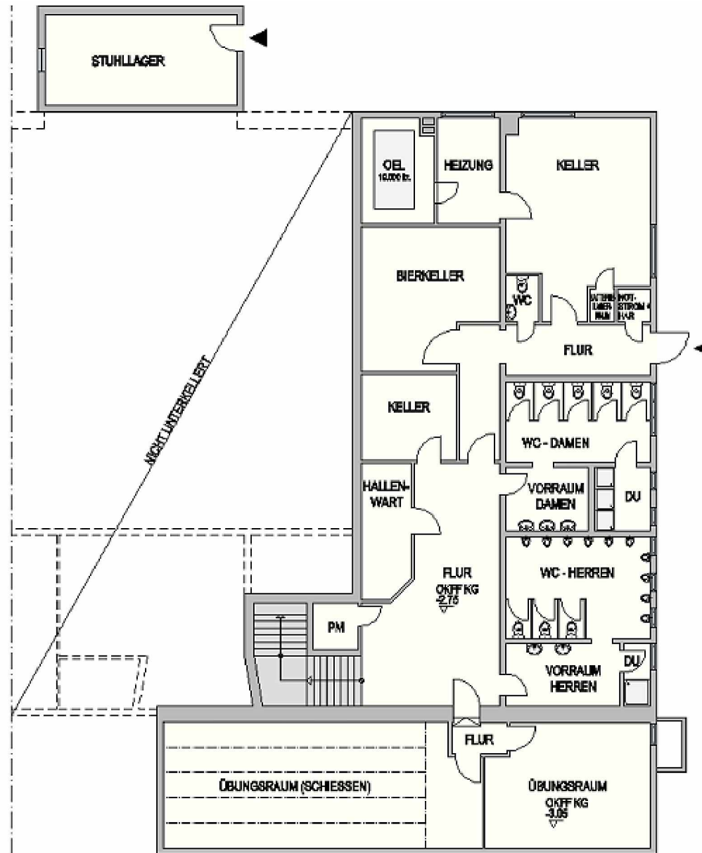
KELLERGESCHOSS
